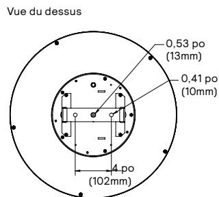
Montage sur tourillon
