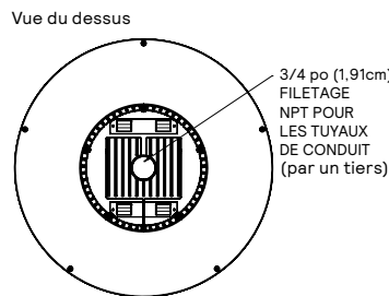
Montage suspendu direct
